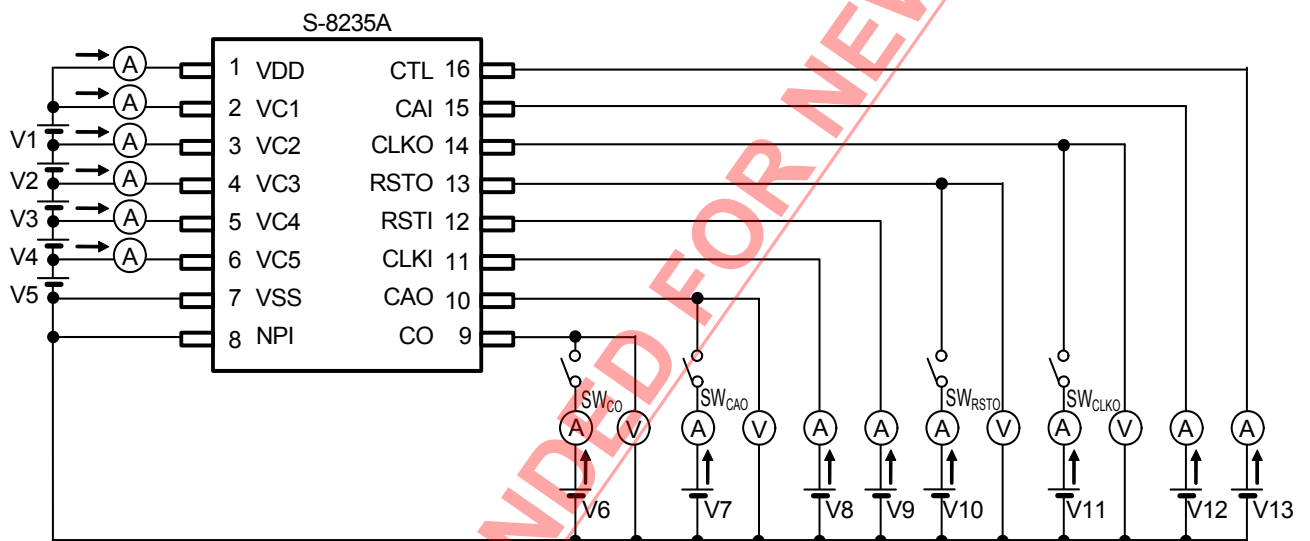
図4 測定回路
