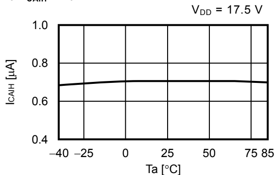
5.10 I_{CAIH} - T_a
