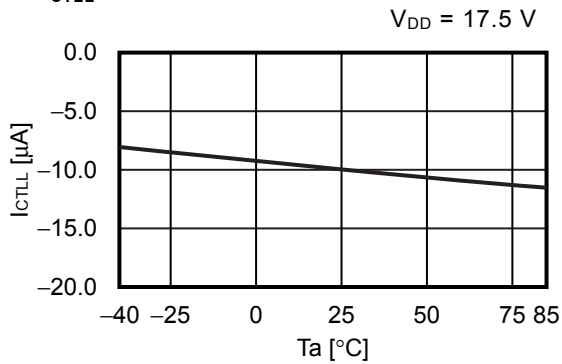
5. 12 I_{CTL L} - T_a
