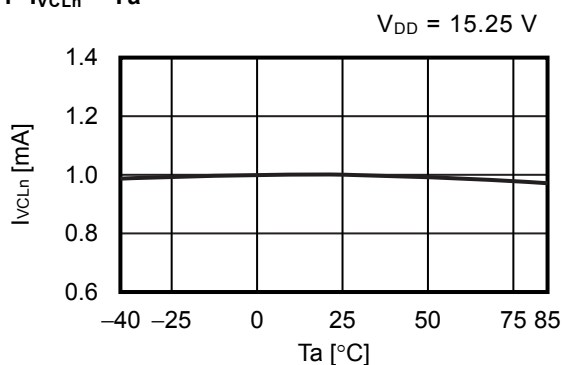
5.1 I_{VCLn} - T_a
