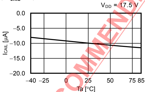
5.9 I_{CAIL} - T_a
