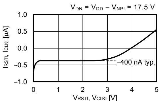
図9 RSTI / CLKI端子電流特性
