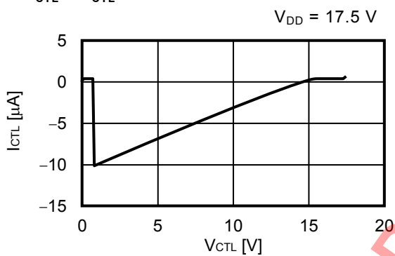
5. 14 I_{CTL} - V_{CTL}
