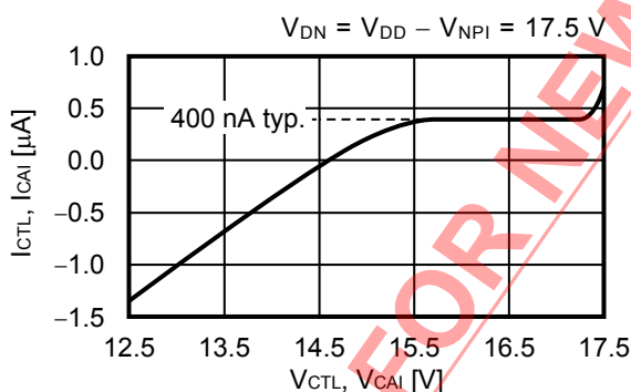
図10 CTL / CAI端子電流特性
