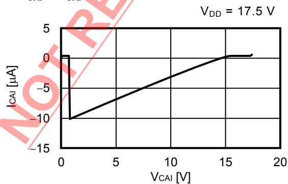
5.11 I_{CAI} - V_{CAI}
