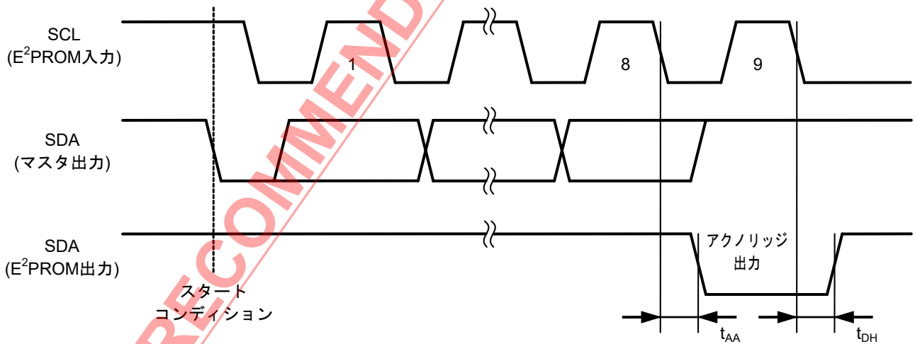
図7 アクノリッジ出力タイミング
