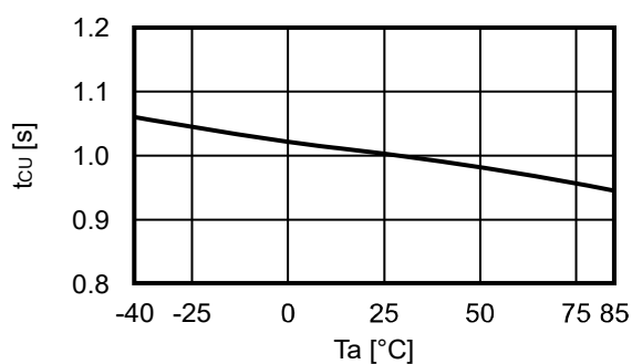
3.1 t_{CU} - T_a
