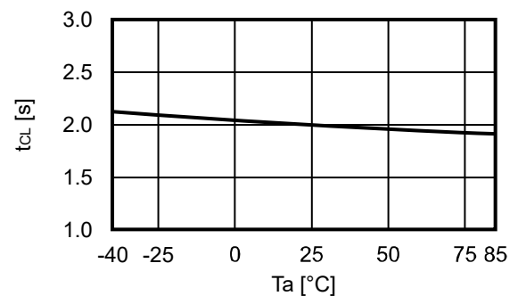
3.2 t_{CL} - T_a
