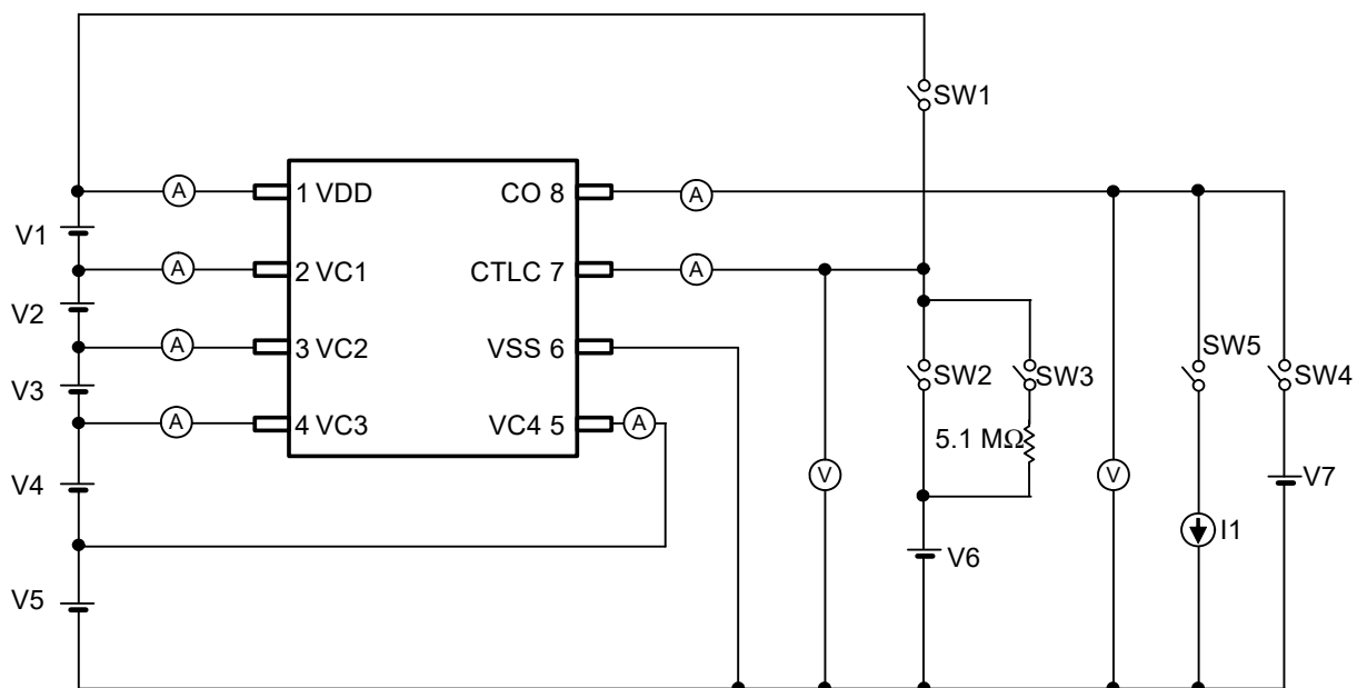
図5 測定回路2
