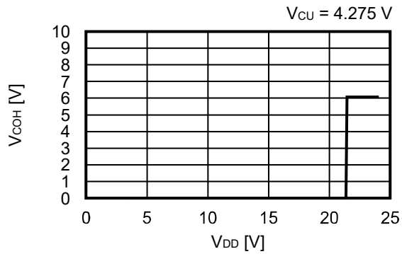
4.3 V_{COH} - V_{DD}
