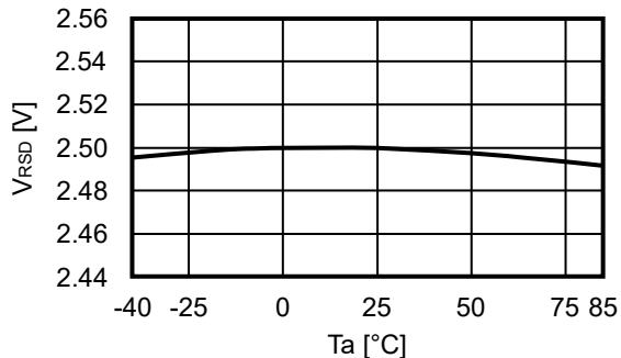
2.3 V RSD – Ta
