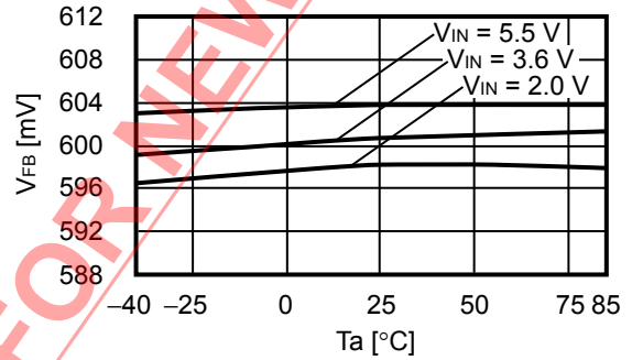
2.10 FB 电压 ( V_{FB} ) — 温度 ( T_a )
