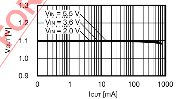
(2) 输出电流 (I OUT ) - 输出电压 (V OUT )
