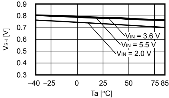
2.7 ON/OFF 端子输入电压“H” ( V_{SH} ) — 温度 ( T_a )
