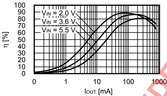
(1) 输出电流 (I OUT ) - 效率 ( \eta )
