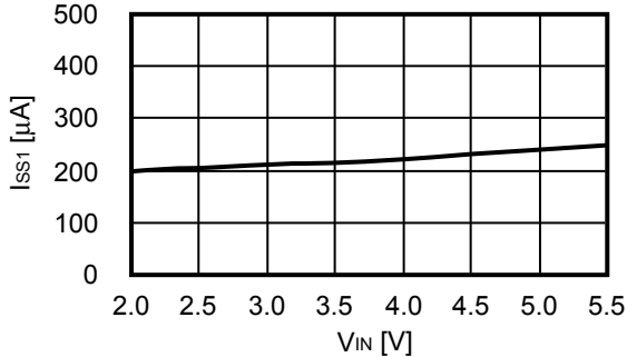
1.1 消耗电流1 (I SS1 ) - 输入电压 (V IN )
