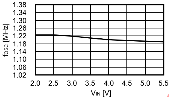
1.3 振荡频率 (f osc ) - 输入电压 (V IN )
