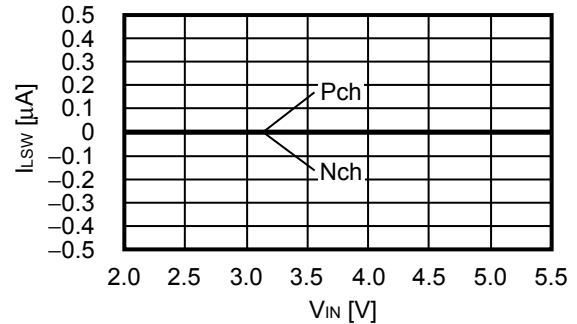
1.6 功率 MOS FET 泄漏电流 (I LSW ) - 输入电压 (V IN )
