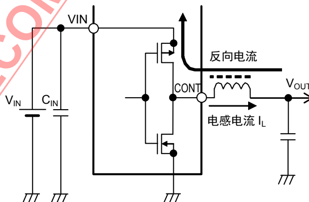
图12 反向电流
