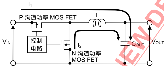
图9 降压型DC/DC控制器的基本电路图
