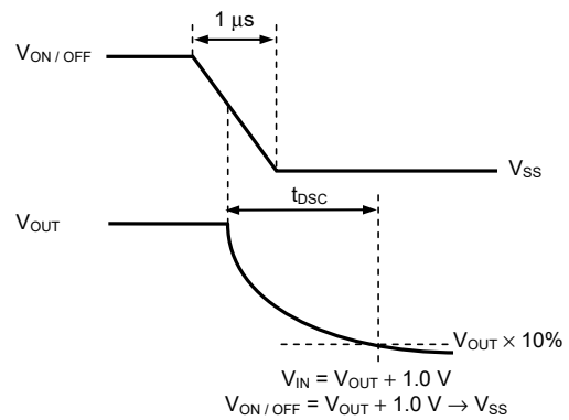
图25 放电时间的测定条件
