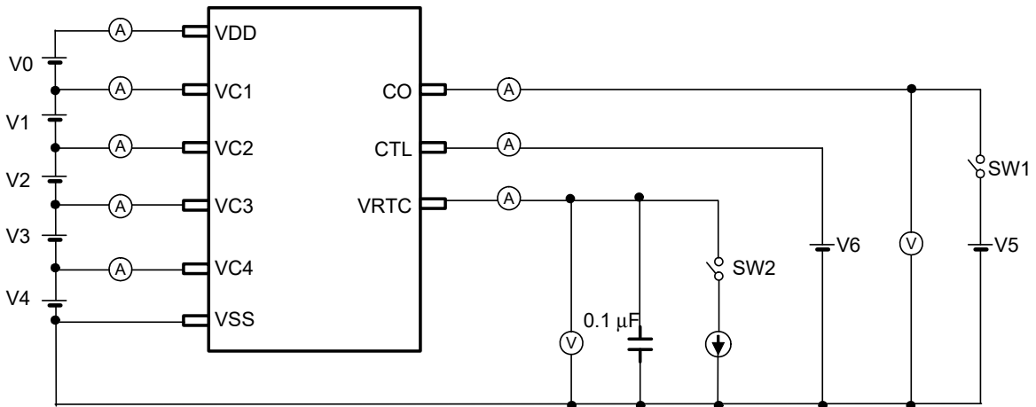
图4 测定电路2
