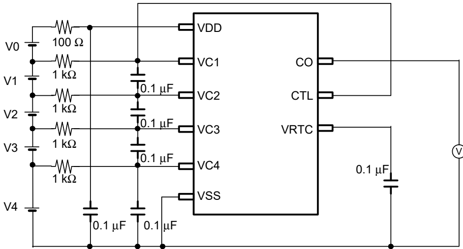
图3 测定电路1
