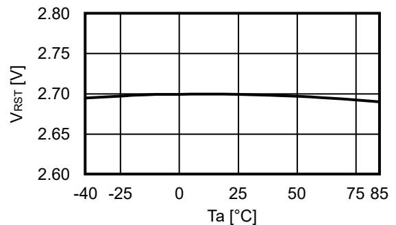
2.4 V_{RST} - T_a
