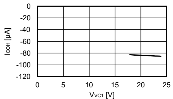
4.2 I_{COH} - V_{VC1}
