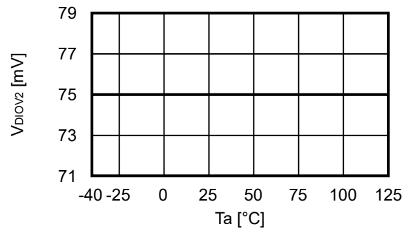
2.8 V_{DIOV2} - T_a
