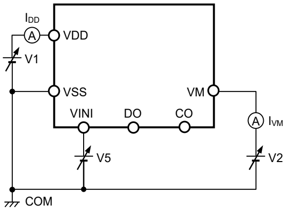
图5 测定电路3
