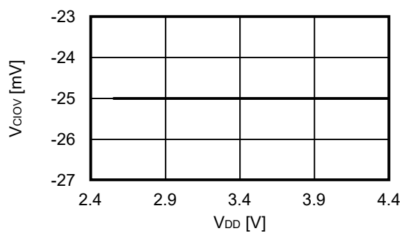
2.11 V_{CI0V} - V_{DD}
