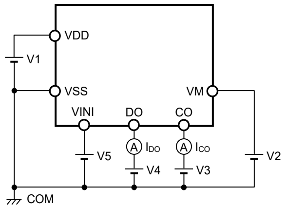
图6 测定电路4
