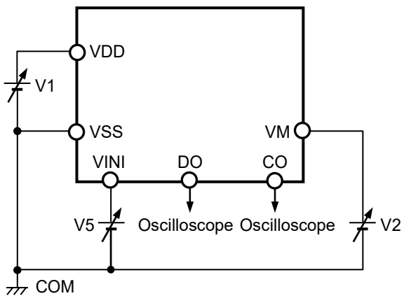
图7 测定电路5
