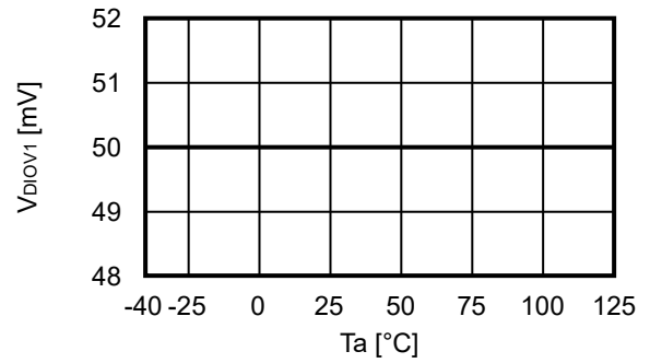
2.6 V_{DIOV1} - T_a
