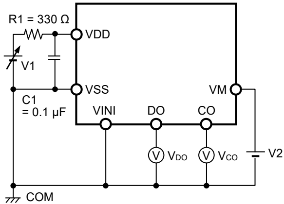
图3 测定电路1
