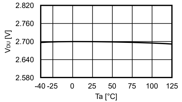
2.4 V_{DU} - T_a
