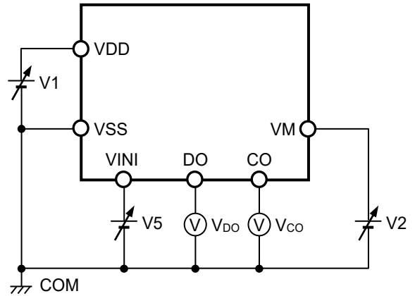
图4 测定电路2
